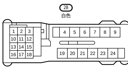
90980-12674
