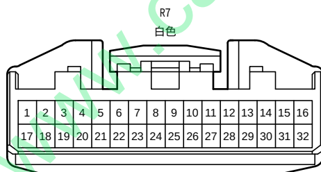
90980-12556
