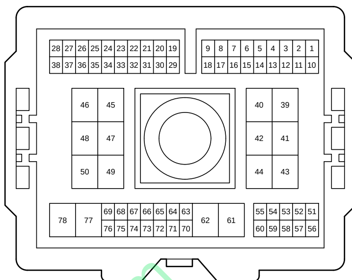
EA3 白色
