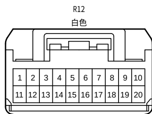
90980-12460
